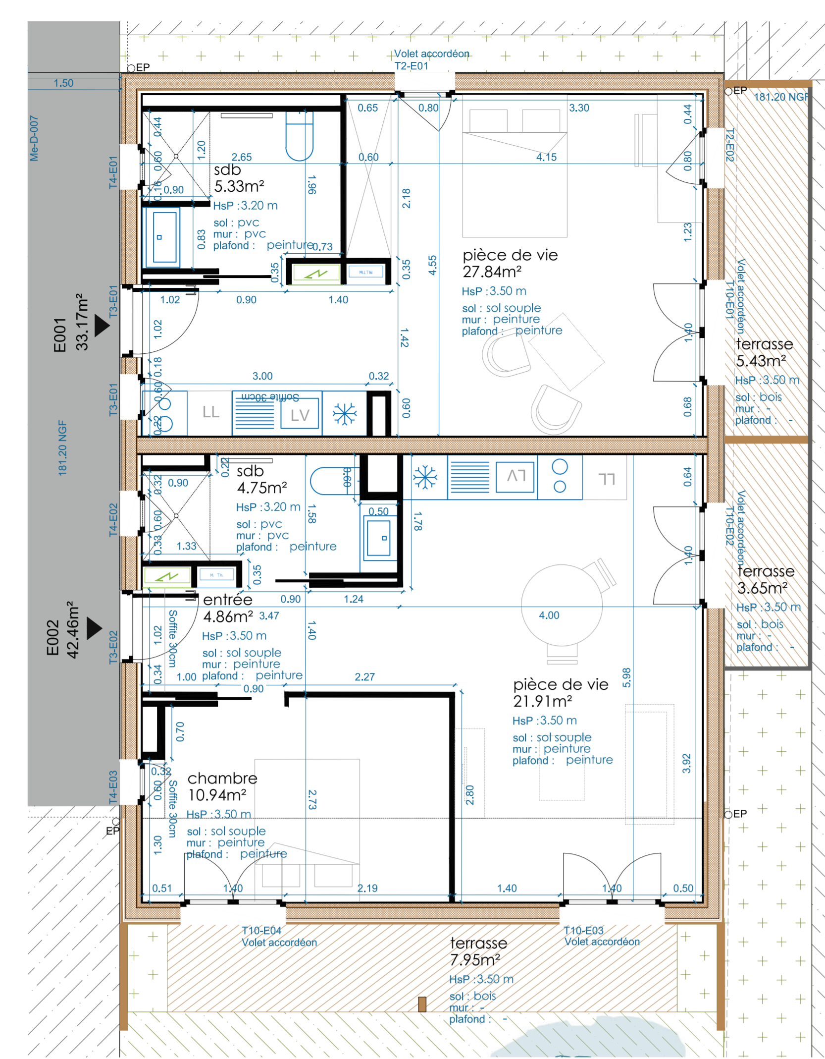
Plan RDC
