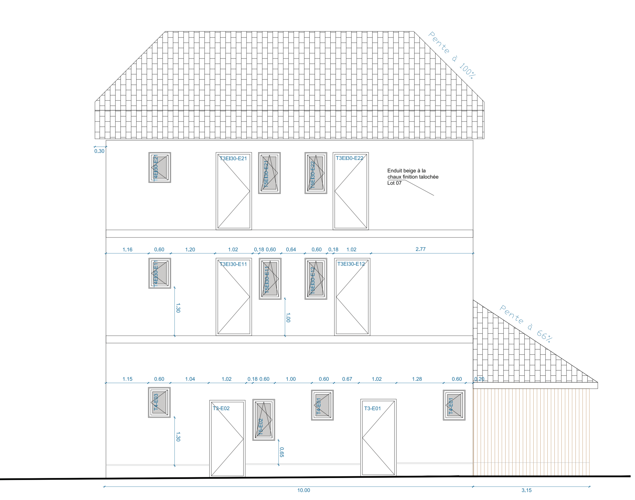
Façades Sud
