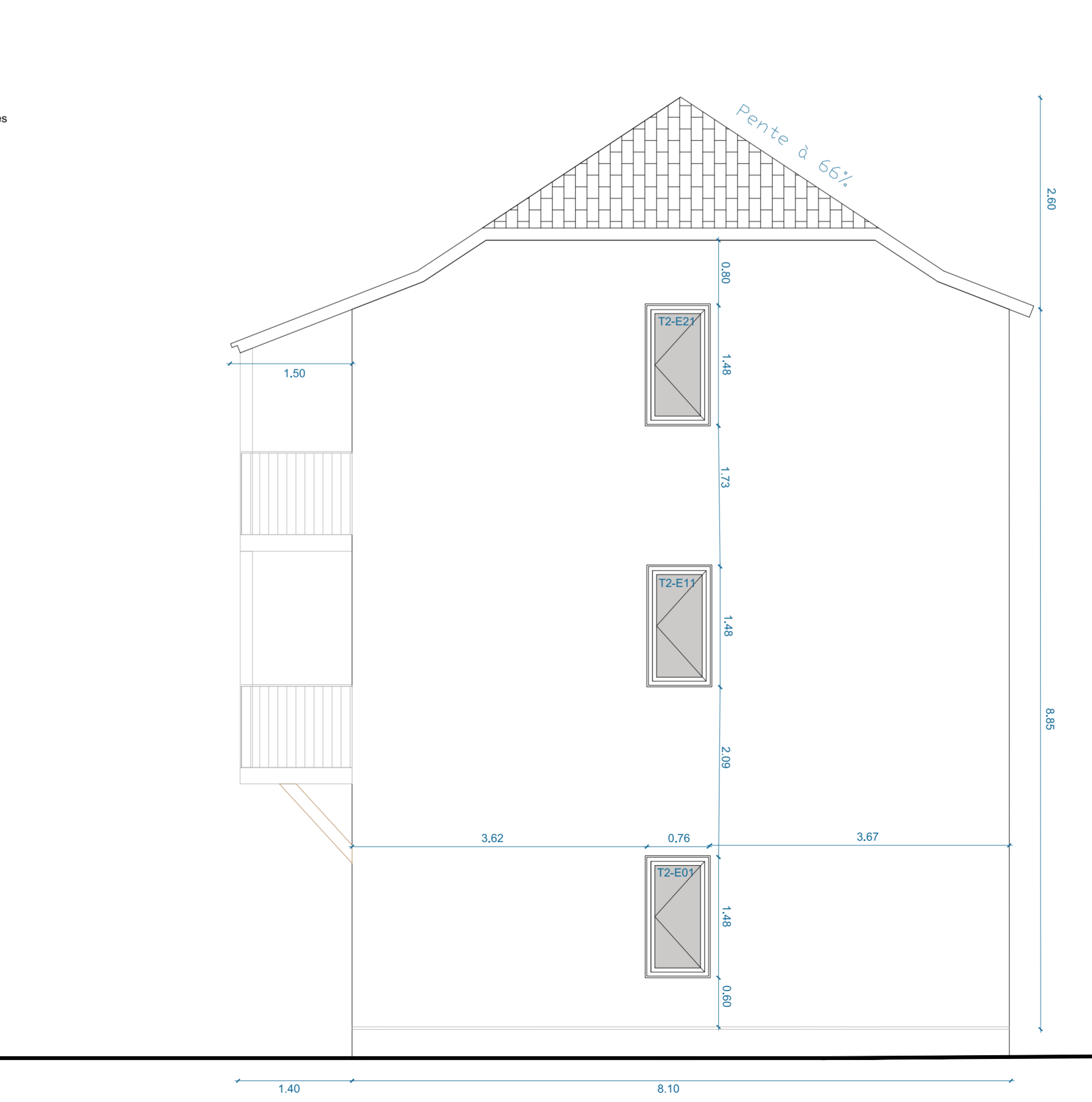
Façades Est
