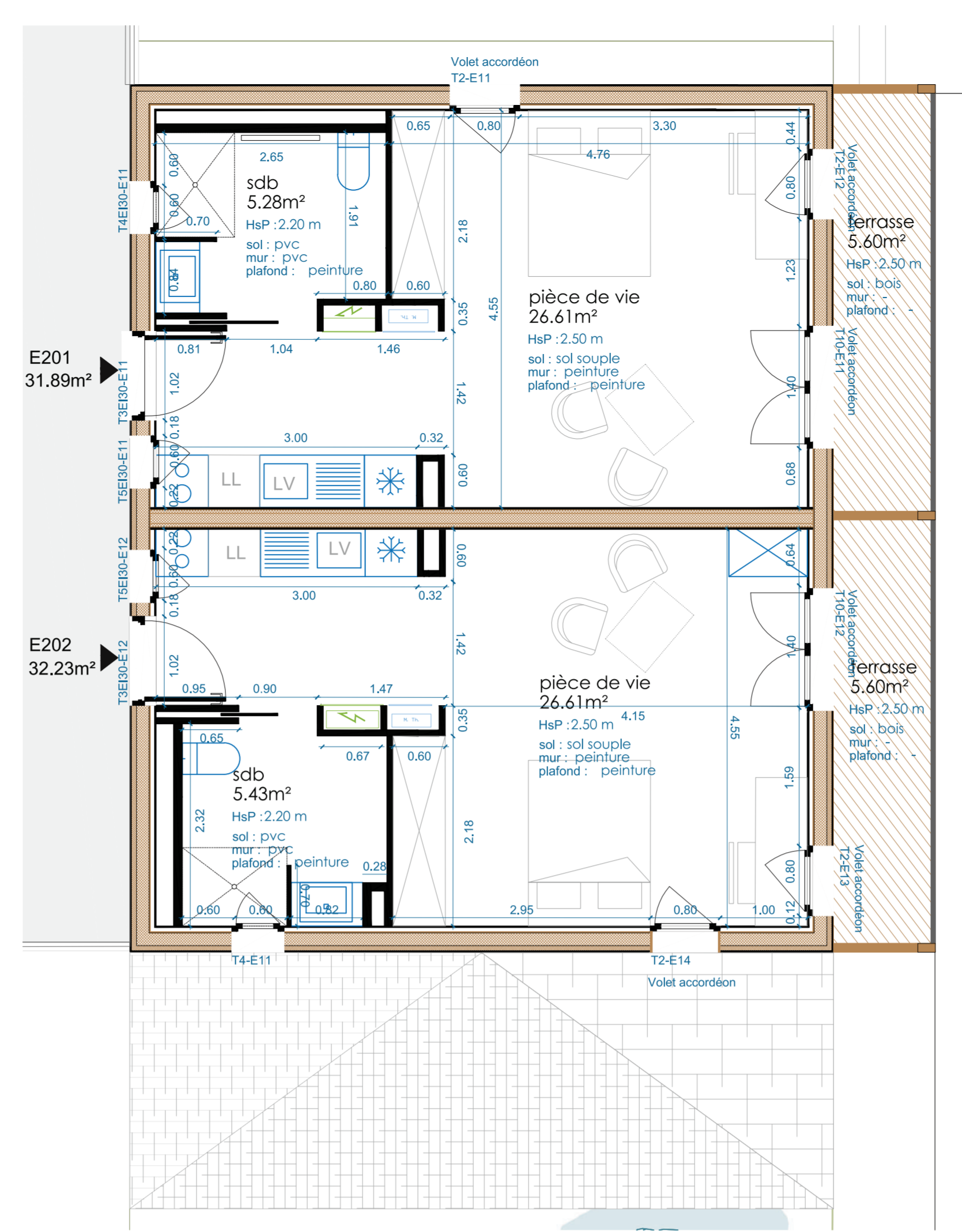
Plan R+2
