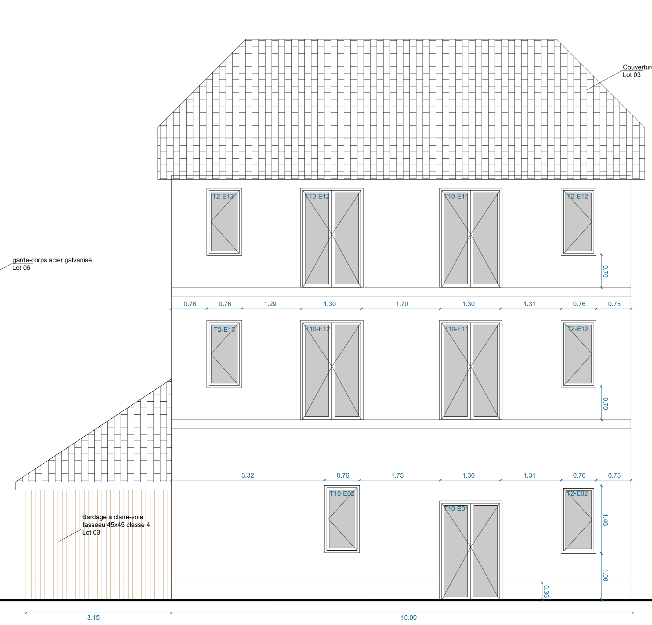
Façades Nord
