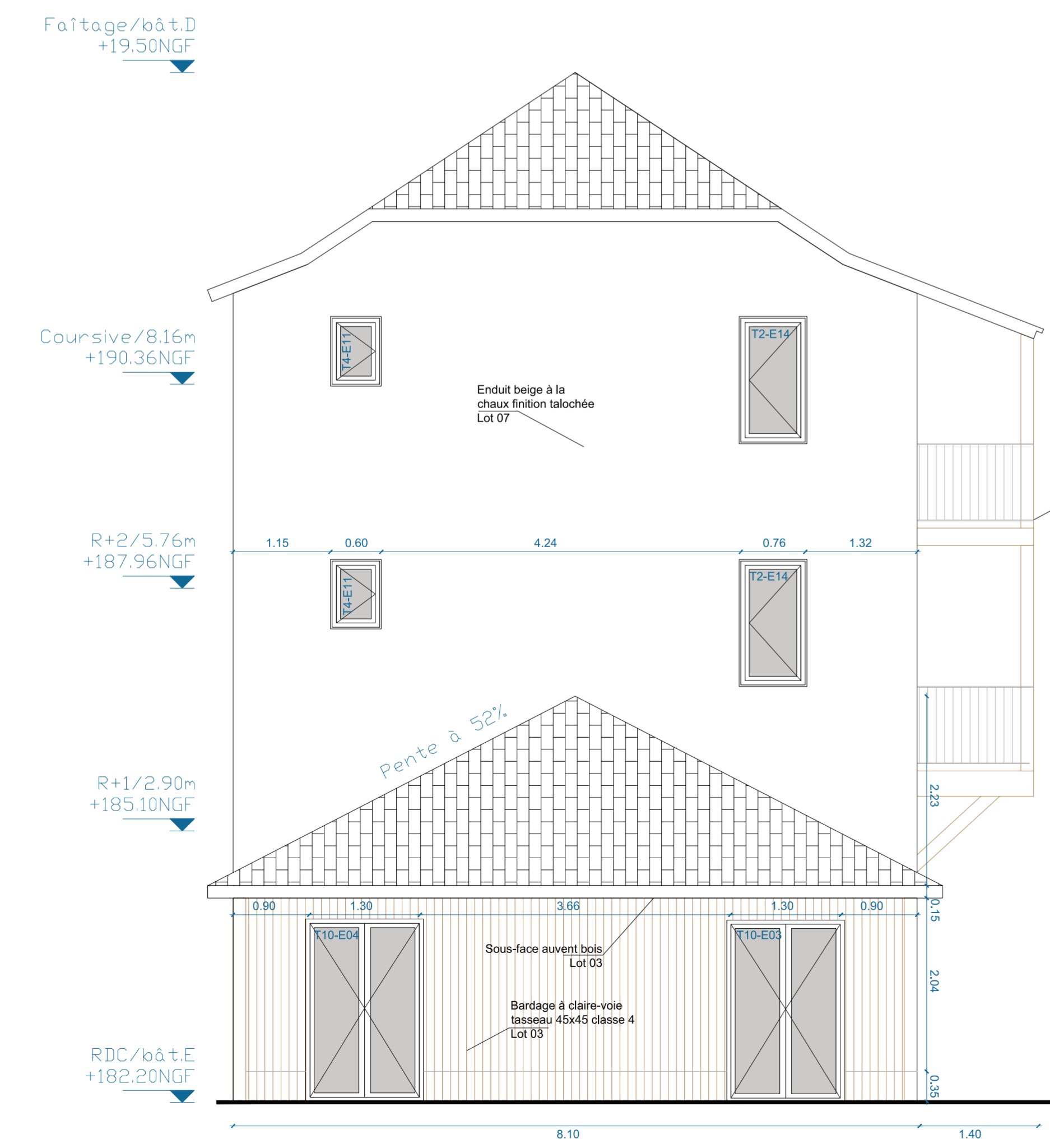
Façades Ouest
